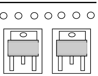
TO252 - 3L
