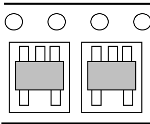
SOT23-5L, TSOT-5L
